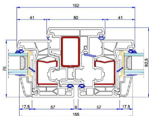
Win Box - nodo centrale simmetrico
