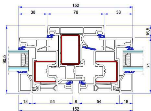
Win Box - nodo centrale simmetrico
