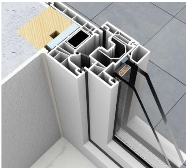
Telaio da ristrutturazione con aletta da 65 mm. Vista telaio completamente in luce.
