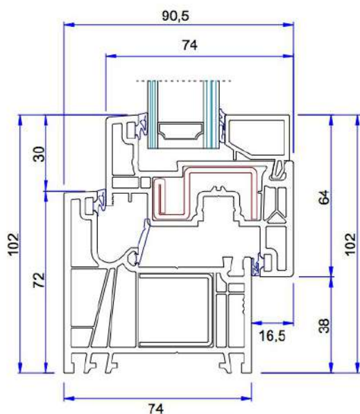
Fermavetro a scatto squadrato
