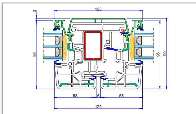
Nodo centrale simmetrico - 123 mm
