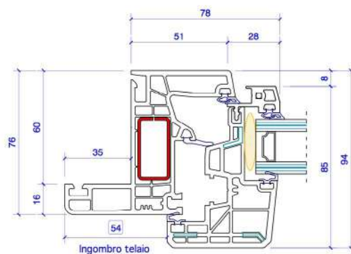
Telaio N con aletta da 35 mm.
