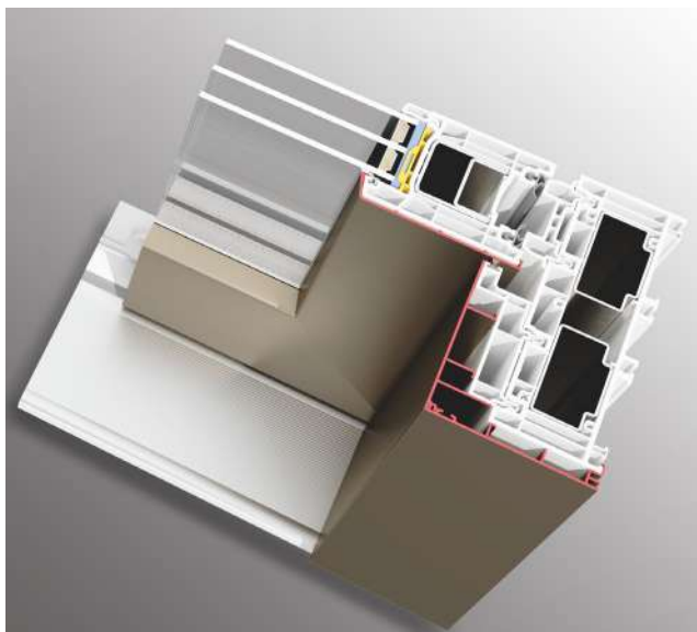
Nodo laterale fisso Minimal.
