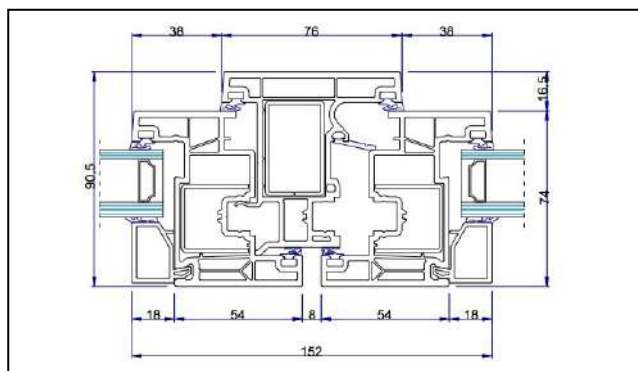
Nodo centrale simmetrico - 152 mm
