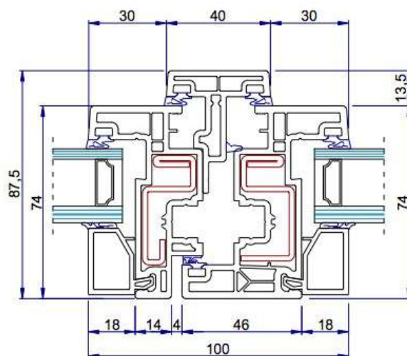
Win Box - nodo centrale asimmetrico
