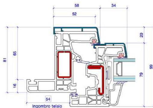
Telaio N con aletta da 35 mm.
