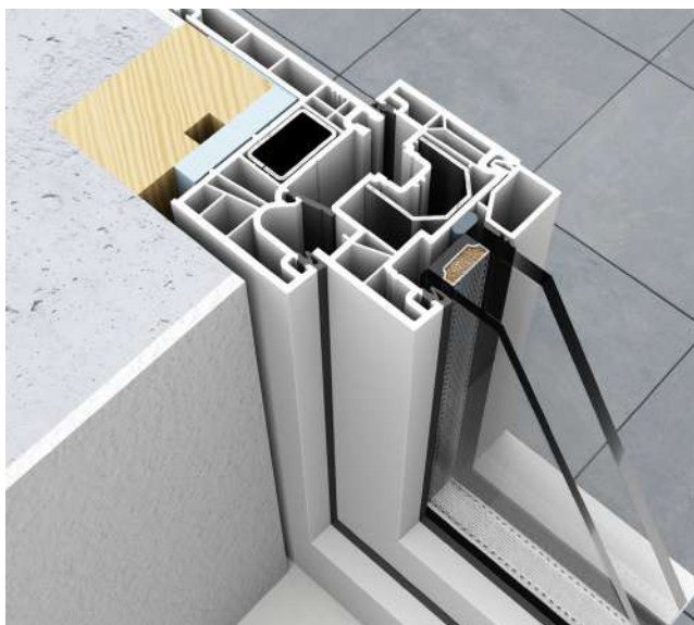
Telaio da ristrutturazione con aletta da 65 mm. Vista telaio parzialmente incassato dietro mazzetta.
