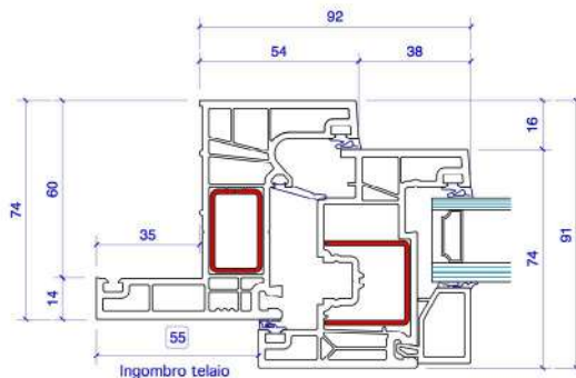
Telaio N con aletta da 35 mm.
