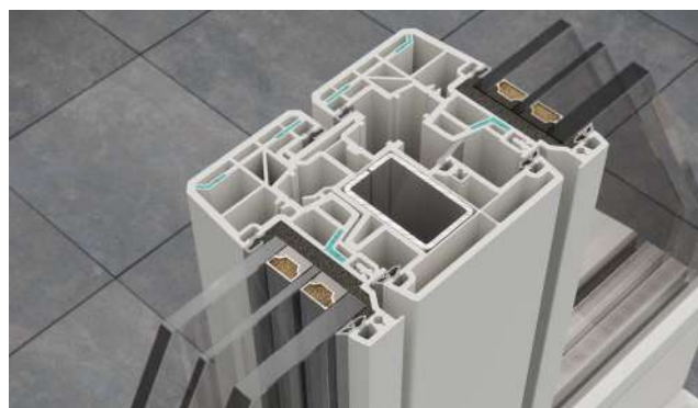
Nodo centrale simmetrico - 125 mm
