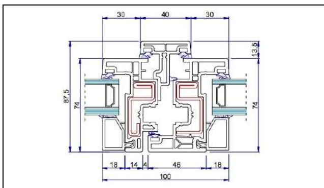
Nodo centrale asimmetrico - 100 mm
