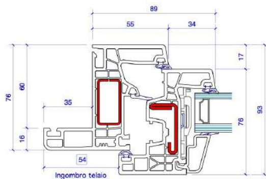
Telaio N con aletta da 35 mm.
