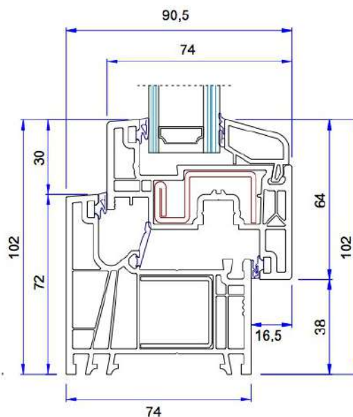
Fermavetro raggio 6 mm stondato
